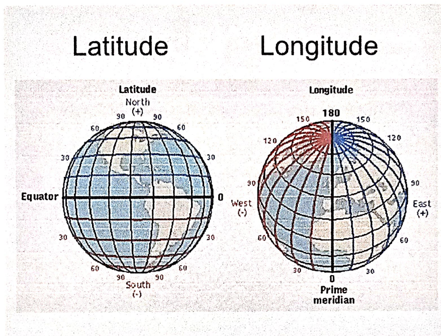
Fig. 4.4 Latitude & Longitude
