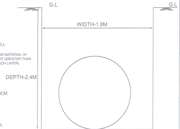
DI PIPE DETAIL (1200 mm)
