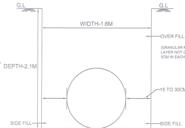
DI PIPE DETAIL (1000 mm)
