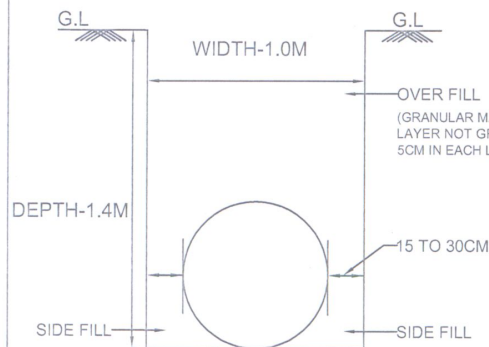
DI PIPE DETAIL (350 MM TO 450MM)
