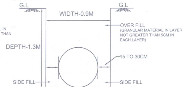
DI PIPE DETAIL (200 MM TO 300MM)
